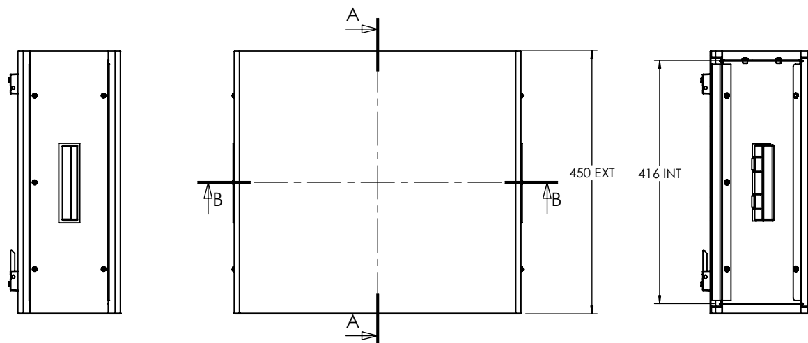
SECTION A-A
